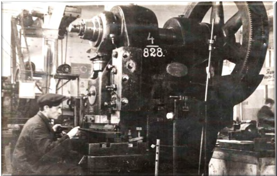
10-тонный механический пресс на фабрике ТАТЯЗМАШ.
