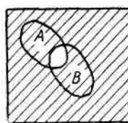
РИС. 9. Операция Шеффера (отрицание конъюнкции \overline{A \wedge B} ).
