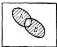
РИС. 8. Отрицание эквивалентности двух высказываний A \not\equiv B
