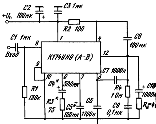
Рис. 2.34. Типовая схема включения ИМС К174УН9 в качестве усилителя мощности. Для установления требуемого коэффициента усиления значения элементов R3 , C4 , C5 могут подбираться
