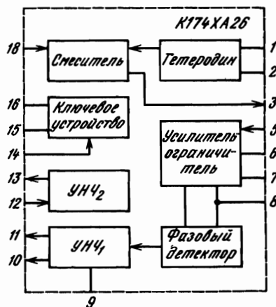
Рис. 2.94. Структурная схема ИМС K174XA26
