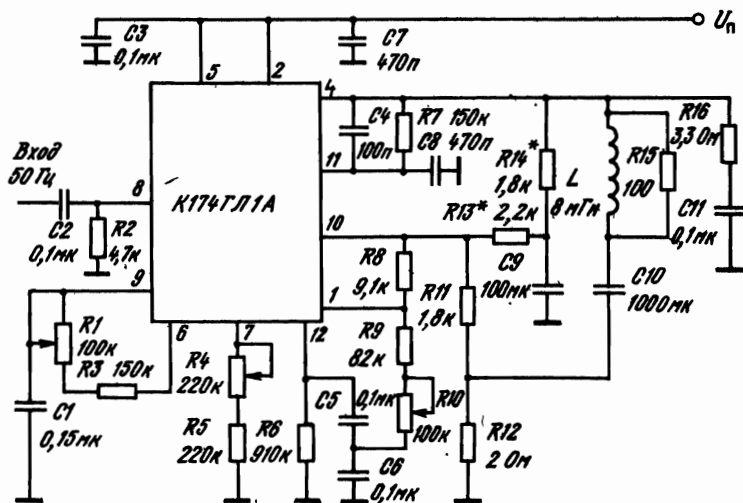
Рис. 2.11. Схема включения ИМС К174ГЛ1, К174ГЛ1А видеомонитора с малым уровнем шума. Сопротивление резистора R6 определяется типом кинескопа и влияет на линейность по вертикали; R15L = 4,5 Ом (отклоняющая система)
