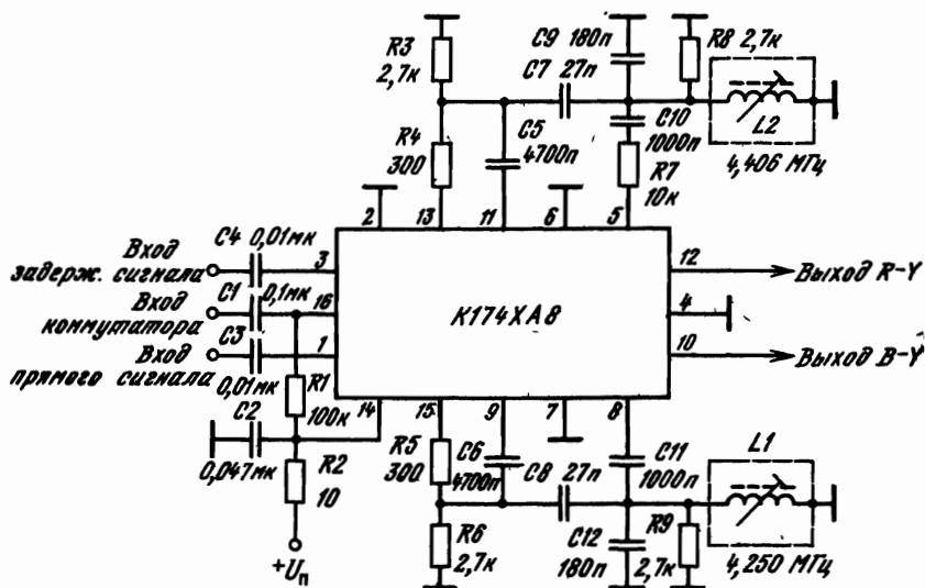
Рис. 2.70. Типовая схема включения ИМС К174ХА8 в качестве электронного коммутатора-демодулятора цветковых сигналов
