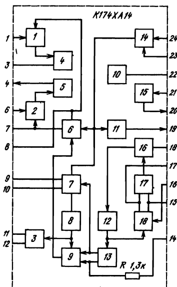
Рис. 2.79. Структурная схема ИМС K174XA14
