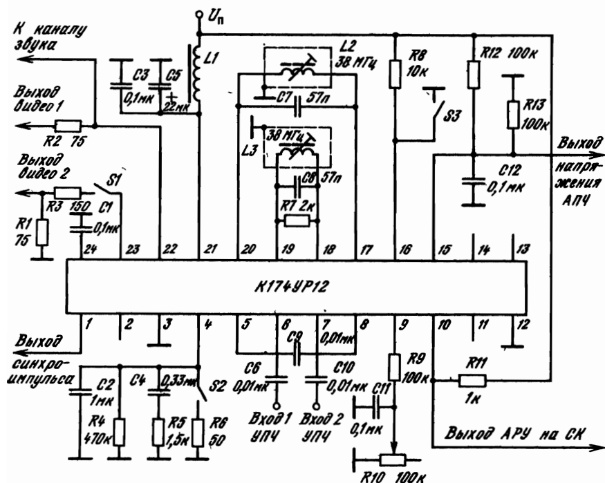
Рис. 2.64. Типовая схема включения ИМС К174УР12 в качестве УПЧ изображений телевизоров
