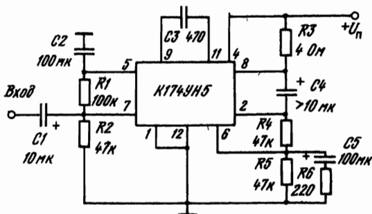
Рис. 2.32. Типовая схема включения ИМС K174УН5 в качестве усилителя мощности
