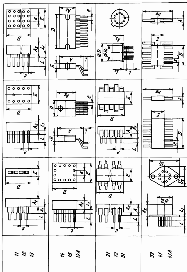
Рис. 1.1. Габаритные чертежи корпусов микросхем
