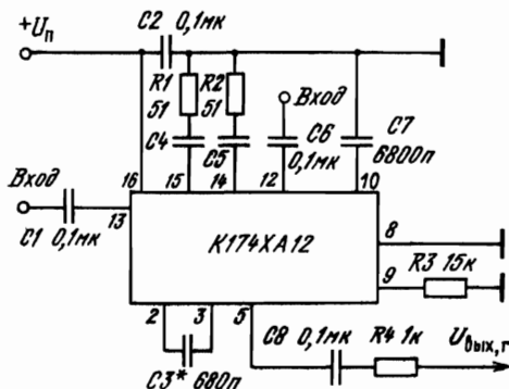
Рис. 2.77 Типовая схема включения ИМС K174XA12 в качестве системы ФАПЧ в режиме следящего фильтра:
