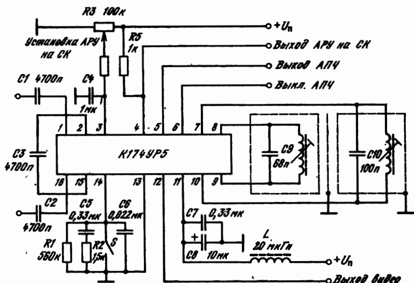
Рис. 2.56. Типовая схема включения ИМС К174УР5 в качестве УПЧ изображения; f_{вх} = 38 \text{ МГц} , Q \geq 50
