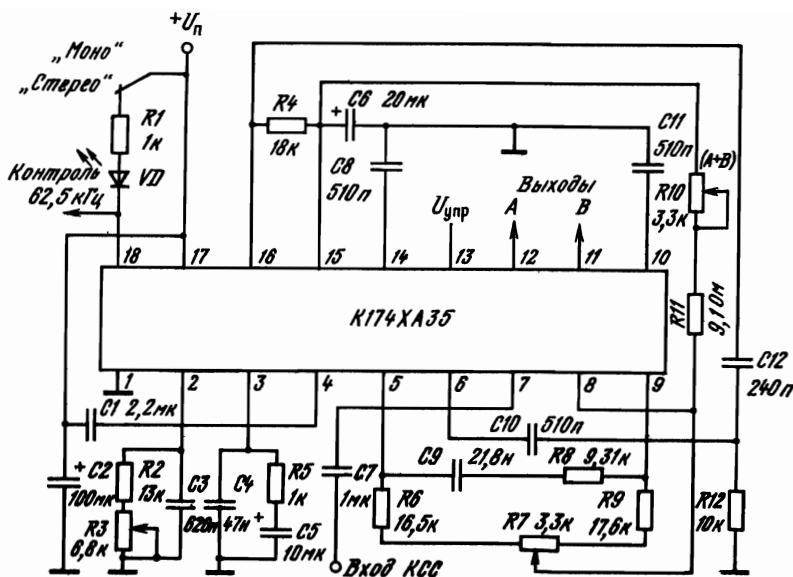
Рис. 2.108. Схема включения ИМС К174ХА35 с подстройкой баланса амплитуд суммарного и разностного сигналов
