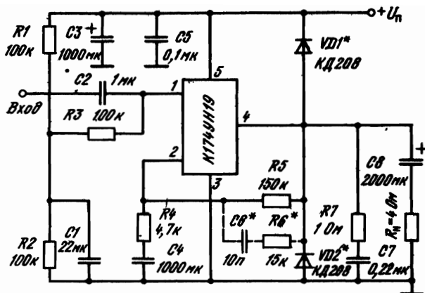
Рис. 2.49. Типовая схема включения ИМС К174УН19 в качестве усилителя мощности с однополярным источником питания при однополярном источнике питания
