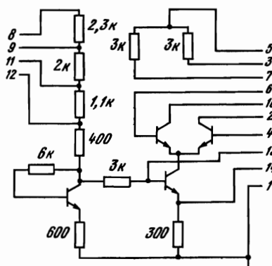
Рис. 2.115. Принципиальная электрическая схема ИМС K175УВ4 (А, Б)
