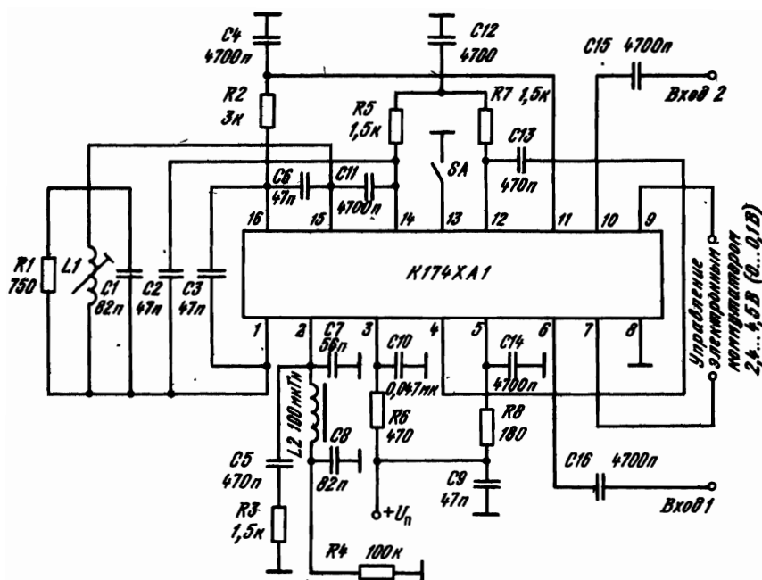
Рис. 2.65. Типовая схема включения ИМС К174ХА1 в качестве синхронного демодулятора цветовой поднесущей телевизоров. Добротность контура L1C1 Q = 50
