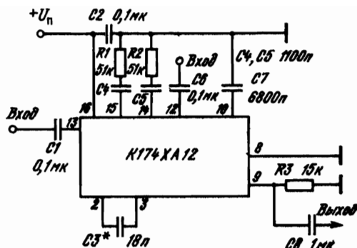
Рис. 2.78. Типовая схема включения ИМС К174ХА12 в качестве системы ФАПЧ в режиме ЧМ-детектора: I_{\text{пот}} = 10 \text{ мА} , K_{\text{АМ}} = 6 \text{ дБ} , C/\text{Ш} = 46 \text{ дБ} при U_{\text{п}} = 18 \text{ В} , f_{\text{вх}} = 10,7 \text{ МГц} , \Delta f = \pm 50 \text{ кГц} , f_{\text{м}} = 1 \text{ кГц}
