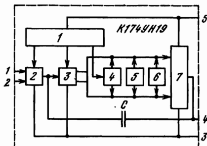
Рис. 2.47. Структурная схема ИМС К174УН19
