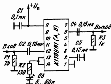
Рис. 2.111. Типовая схема включения ИМС K175УВ1 (А, Б) в качестве широкополосного УВЧ. Выводы 3, 4 и 5 от вспомогательного автономного n-p-n транзистора служат для расширения функциональных возможностей микросхемы [4]
