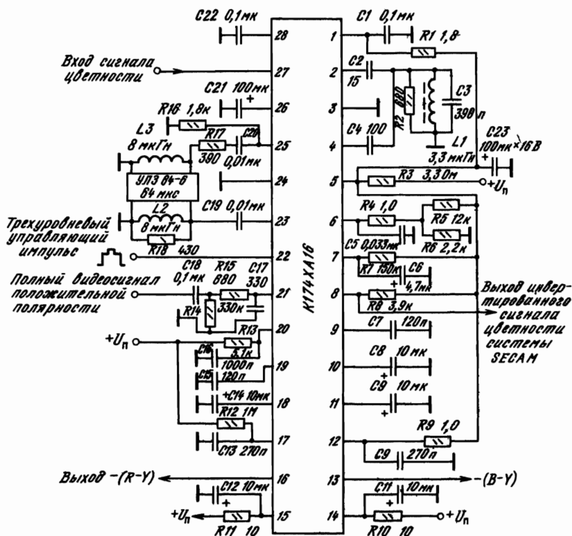
Рис. 2.84. Типовая схема включения ИМС К174ХА16 в качестве декодера цветных сигналов телевизоров
