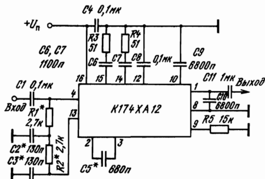
Рис. 2.76. Типовая схема включения ИМС K174XA12 в качестве системы ФАПЧ в режиме синхронного АМ-детектора:
