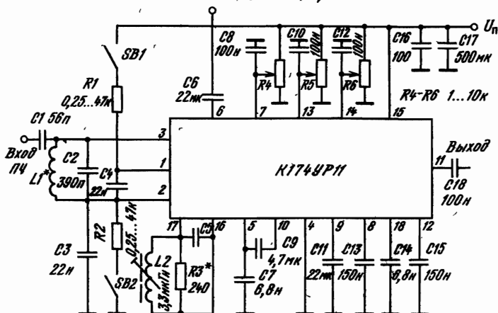
Рис. 2.62. Типовая схема включения ИМС К174УР11 в качестве УПР каналов звука с электронной регулировкой тембра: L2 — 3,3 мкГн, сердечник МР-2СБ-126
