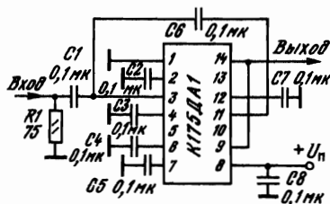
Рис. 2.110. Типовая схема включения ИМС K175ДА1 в качестве детектора АМ-сигналов [4]
