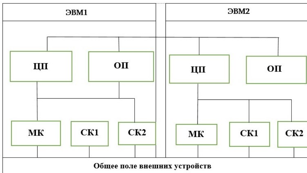
Рис. 1. Структурная схема СВК (ЦП – центральный процессор, МК – мультиплексный канал, СК – селекторный канал, ОП – оперативный канал)
