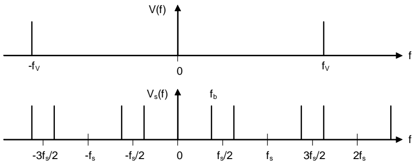
Рис. 2 – Отражения при дискретизации действительного сигнала
