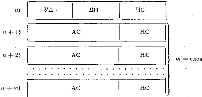
РИС. 26. Ассоциативный узел.
