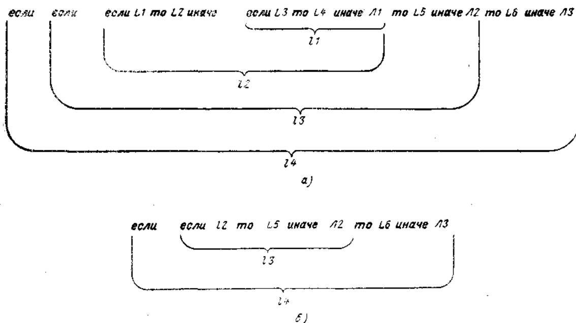
РИС. 13. Пример условного логического выражения: а — исходное выражение; б — после первого этапа преобразования.
