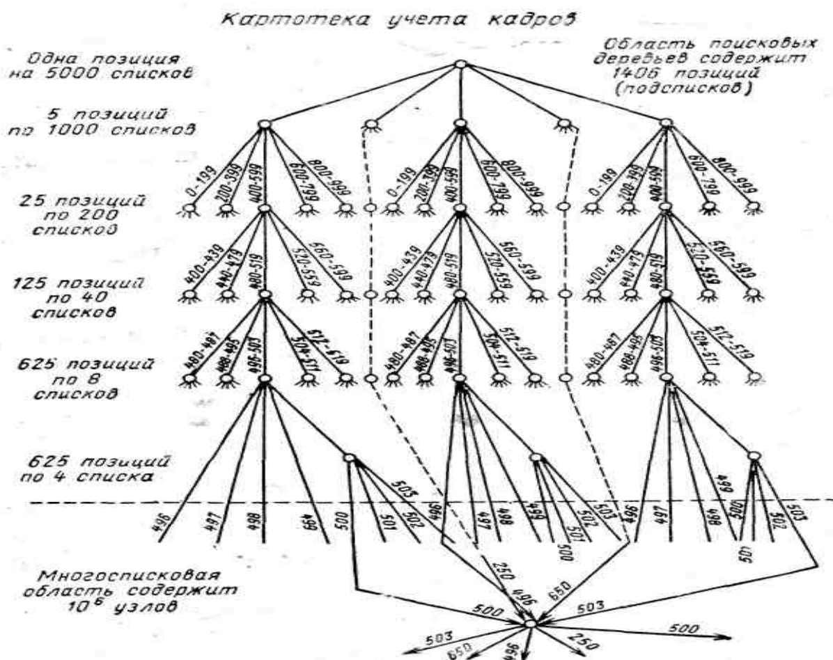
РИС. 18. Многосписковая структура.
