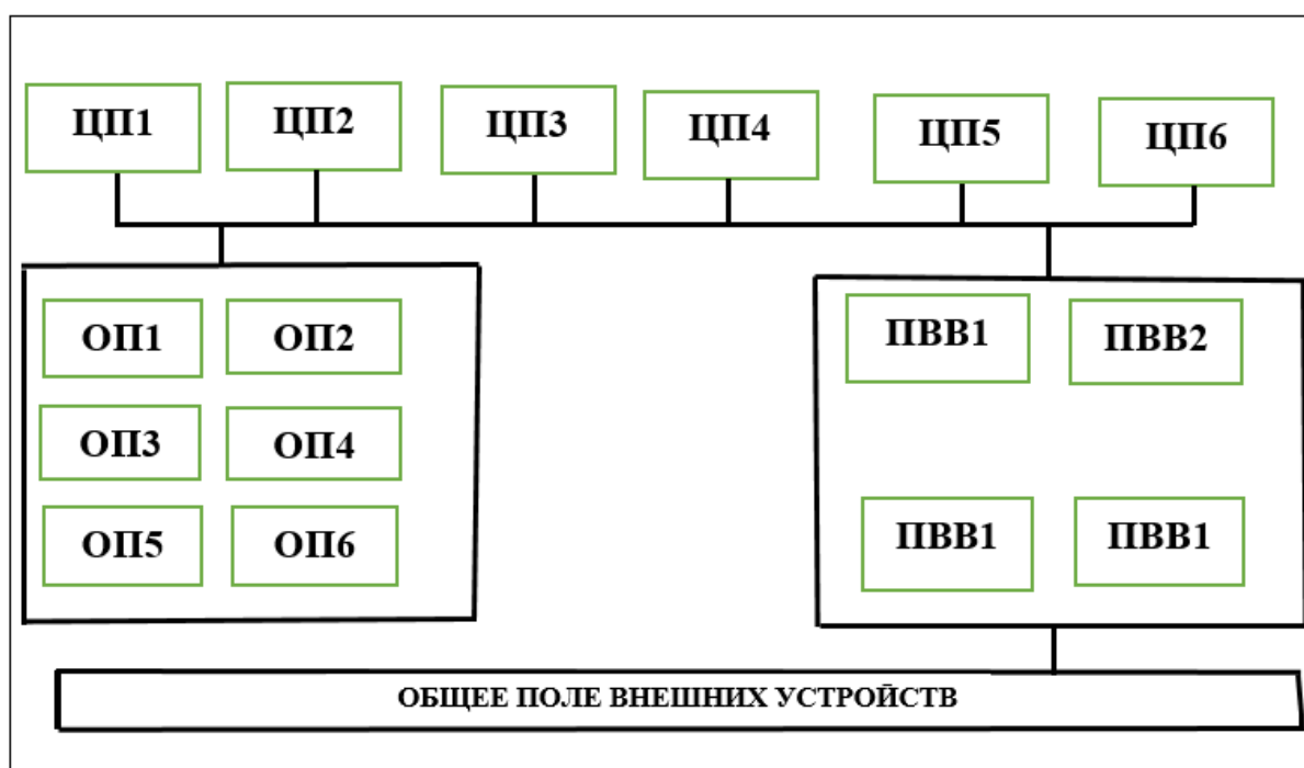
Рис. 1. Структурная схема ВК «Севан» (ЦП – центральный процессор, ПВВ – процессор ввода-вывода, ОП – оперативный канал)
